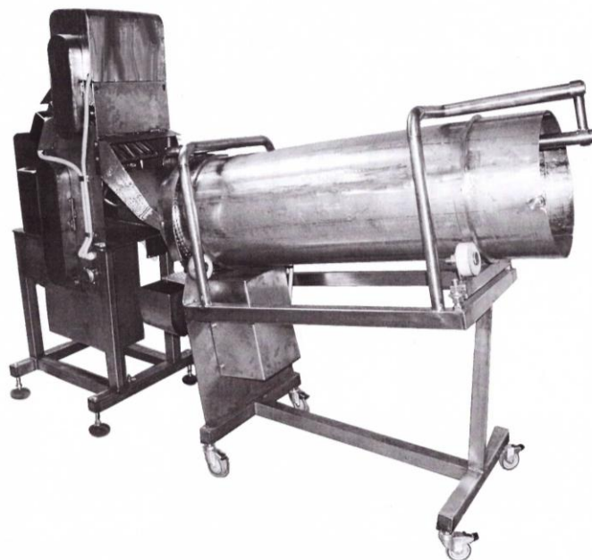
Устройство для разделки полутушек птицы на части
